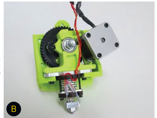
LulzBot Flexystruder
